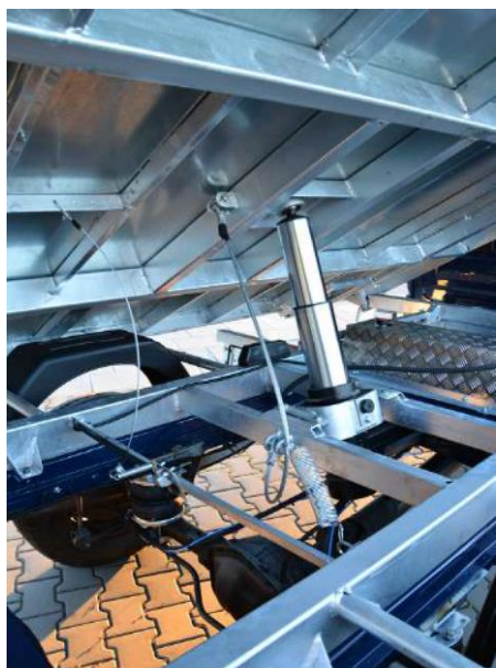
Zdvihací píst a bezpečnostní podpěra zvednuté korby
